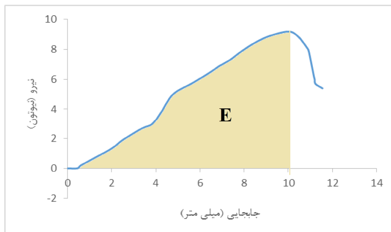
شکل ۳: نمودار نیرو - جابجایی ثبت شده با دستگاه آزمون
