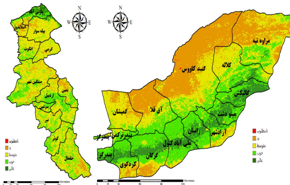
شکل ۱۰- پهنه‌بندی نهایی گلستان و اردبیل
