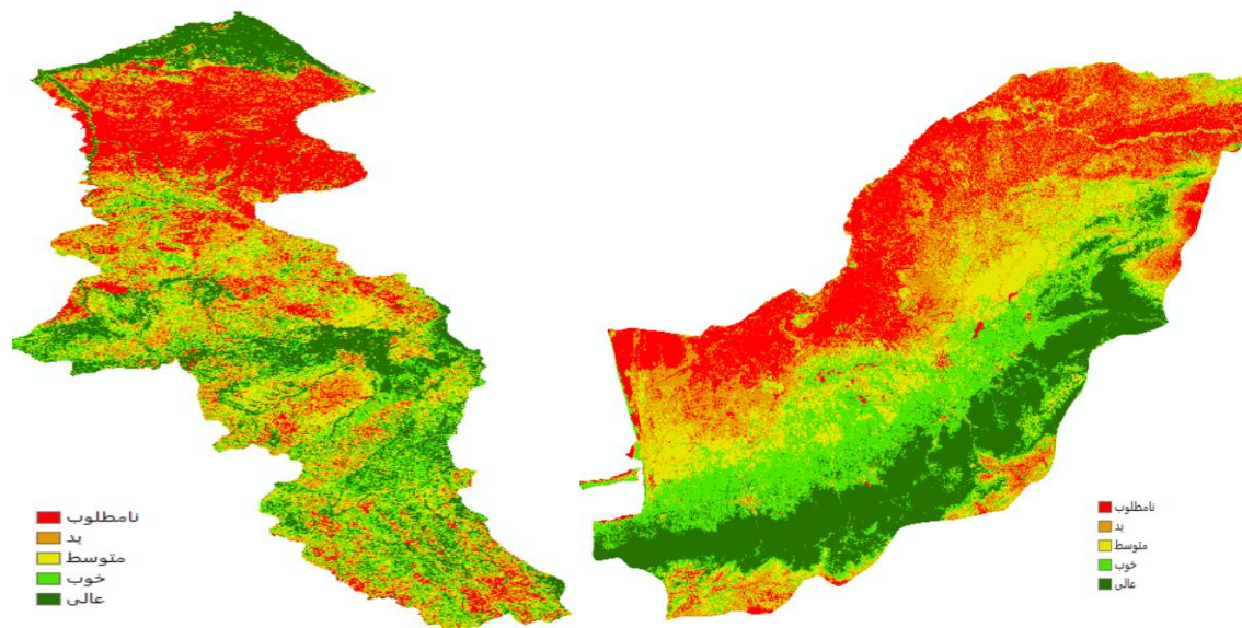
شکل ۸- طبقه بندی NDSI خاک گلستان و اردبیل
