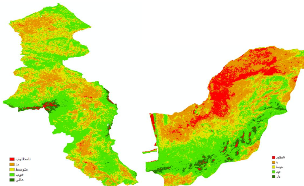
شکل ۶- طبقه بندی PH گلستان و اردبیل
