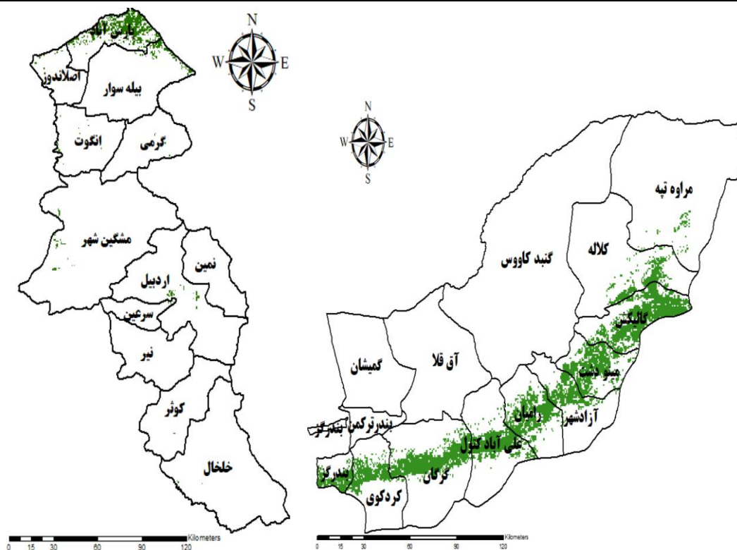
شکل ۱۱- مناطق عالی جهت کشت پنبه گلستان و اردبیل
