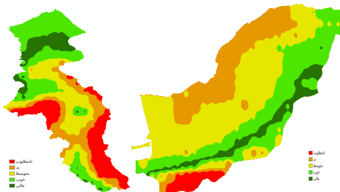
شکل ۷- طبقه بندی دمای خاک گلستان و اردبیل
