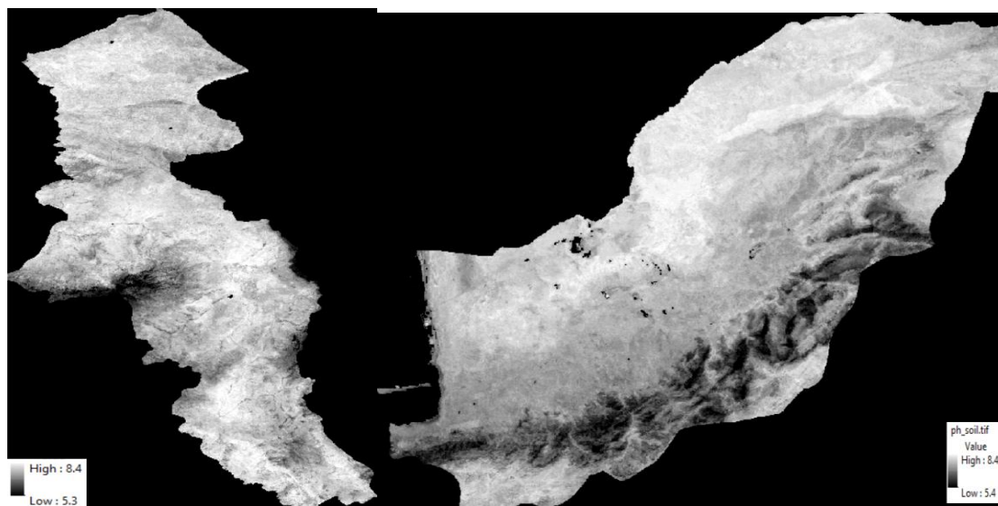
شکل ۲- نقشه pH گلستان و اردبیل
