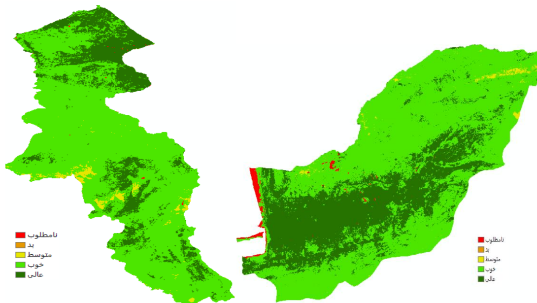
شکل ۹- طبقه بندی بافت خاک گلستان و اردبیل
