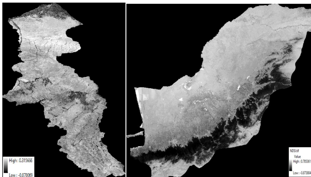
شکل ۴- NDSI گلستان و اردبیل
