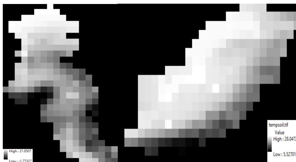
شکل ۳- نقشه دمای خاک سه ماهه اول گلستان و اردبیل
