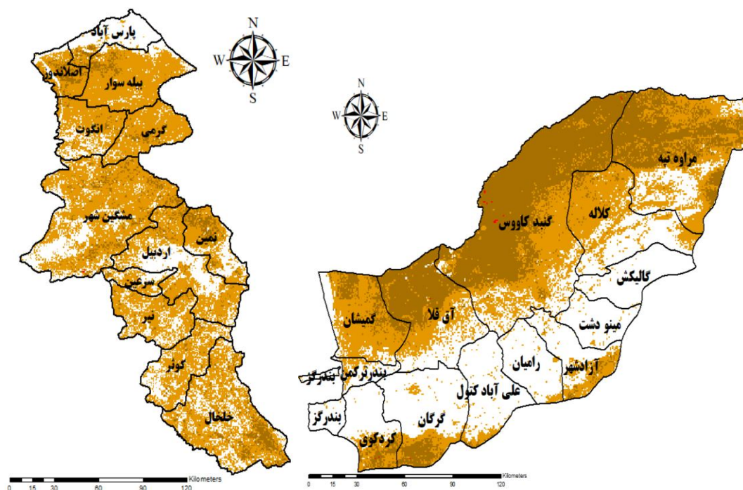
شکل ۱۲- مناطق بد جهت کشت پنبه گلستان و اردبیل
