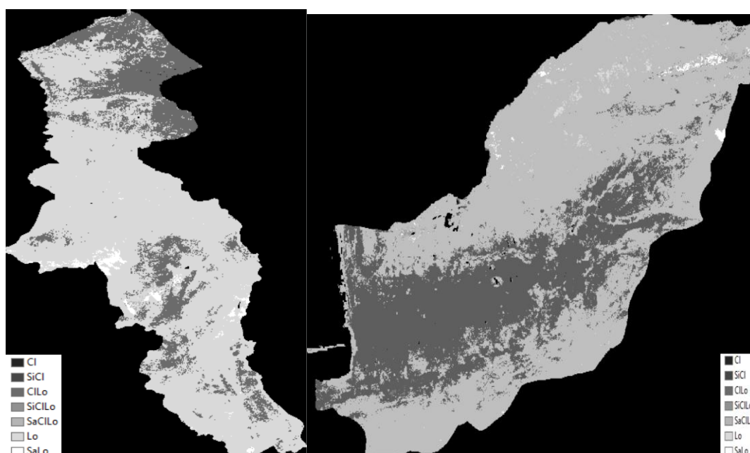
شکل ۵- بافت خاک گلستان و اردبیل
